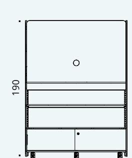
Vue de face Support TV
